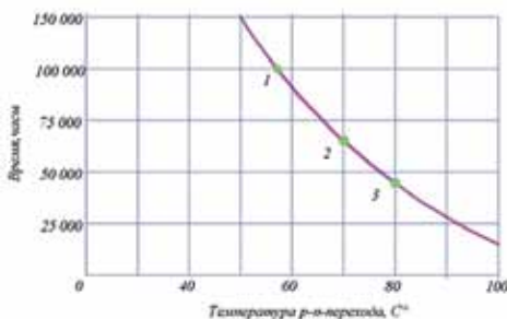
Рисунок 4. Зависимость срока службы светодиодов до уменьшения светового потока на 50% от температуры на кристалле
