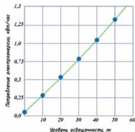
Рисунок 2. Зависимость потребления электроэнергии системой светодиодного освещения ИСО «Хамелеон» от уровня освещенности при высоте подвеса 3 м для светильников СН1050-12-60-Х цветовой температуры 5500 К
